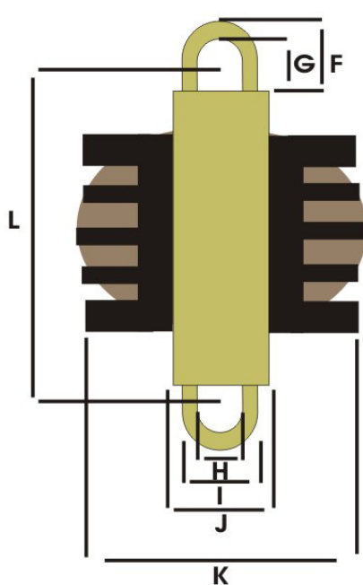
VISTA SUPERIOR
